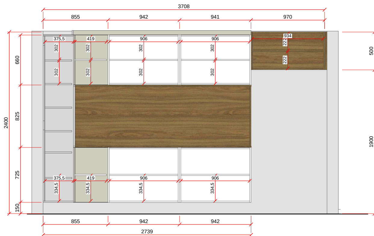
VISTA C - ESC. 1:30
